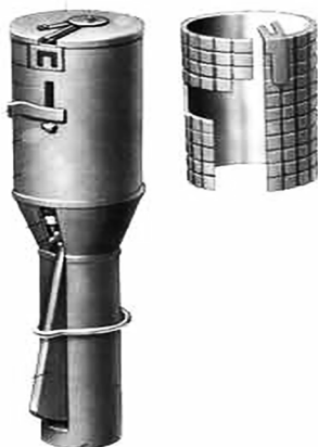
Русская ручная граната, времен Первой мировой войны (от 200 до 300 осколков, с чехлом до 1000 осколков)
