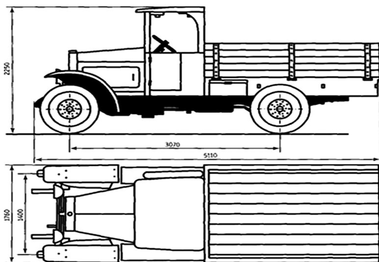
Схема автомобиля АМО-Ф-15
